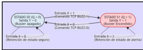
FIGURA 4. MODELO DE MÁQUINA DE ESTADOS FINITOS (TIPO MOORE) PARA EL CIRCUITO ACTUADOR: CONTROL DE TRANSICIONES BINARIAS (Q) Y SALIDAS FÍSICAS (Y) MEDIADAS POR COMANDOS DE RED (X).
