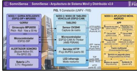
FIGURA 1. DIAGRAMA DE BLOQUES DEL SISTEMA DISTRIBUIDO DE ALERTA DE FATIGA: ORGANIZACIÓN DE LOS NODOS PORTÁTIL, CENTRAL Y DE PROCESAMIENTO MÓVIL, MÓDULOS DE REPORTE E INTELIGENCIA ARTIFICIAL, INTERFACES DE COMUNICACIÓN INALÁMBRICA Y PERIFÉRICOS DE SALIDA FÍSICA.
