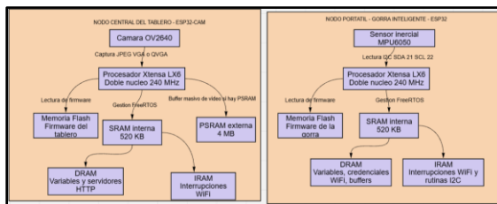
FIGURA 3. DISTRIBUCIÓN LÓGICA DEL MAPA DE MEMORIA MULTIPLEXADO ENTRE AMBOS NODOS DEL SISTEMA.
