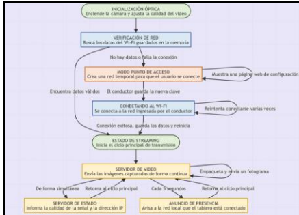
FIGURA 6. MÁQUINA DE ESTADOS FINITOS DEL NODO CENTRAL DEL TABLERO.
